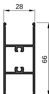
H-635 kg/m 0.853
