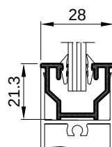
H-638 kg/m 0.291
