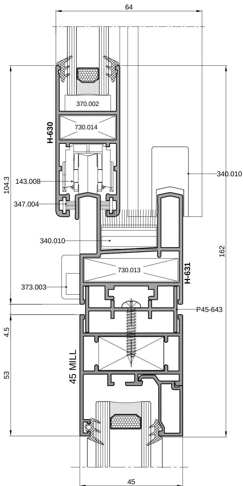
Spoj serije Harmo (dvostazno) sa serijom 45 Mill
