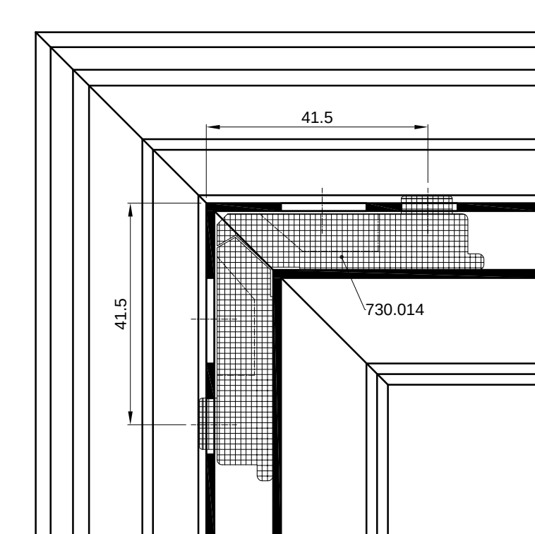
PRESJEK A-A
