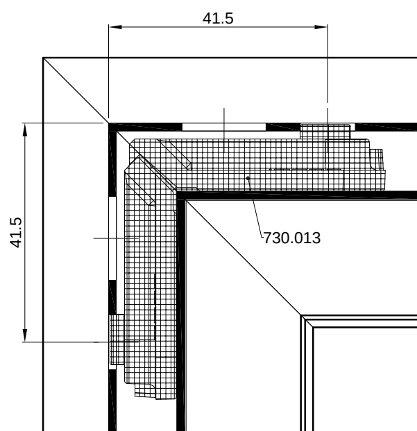
PRESJEK A-A
