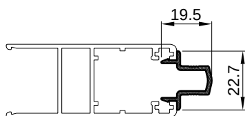
H-637 kg/m 0.210
