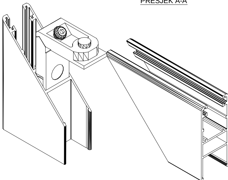
PRESJEK A-A
