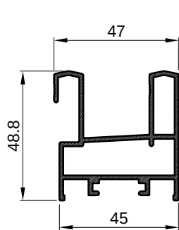
H-631 kg/m 1.033
