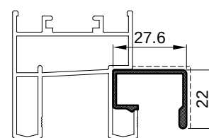
H-636 kg/m 0.277
