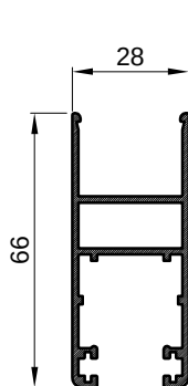
H-630 kg/m 0.861
