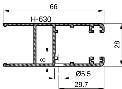
Presjek A-A
